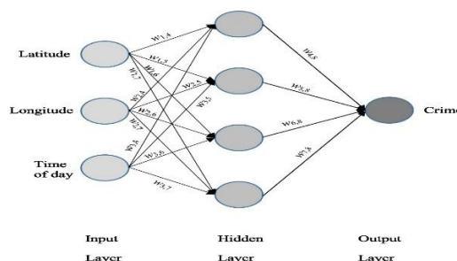
Схема 1. Образец контролируемого обучения ANN [Многослойный персептрон (MLP)] для прогнозирования типа преступления по данным о времени и месте.
